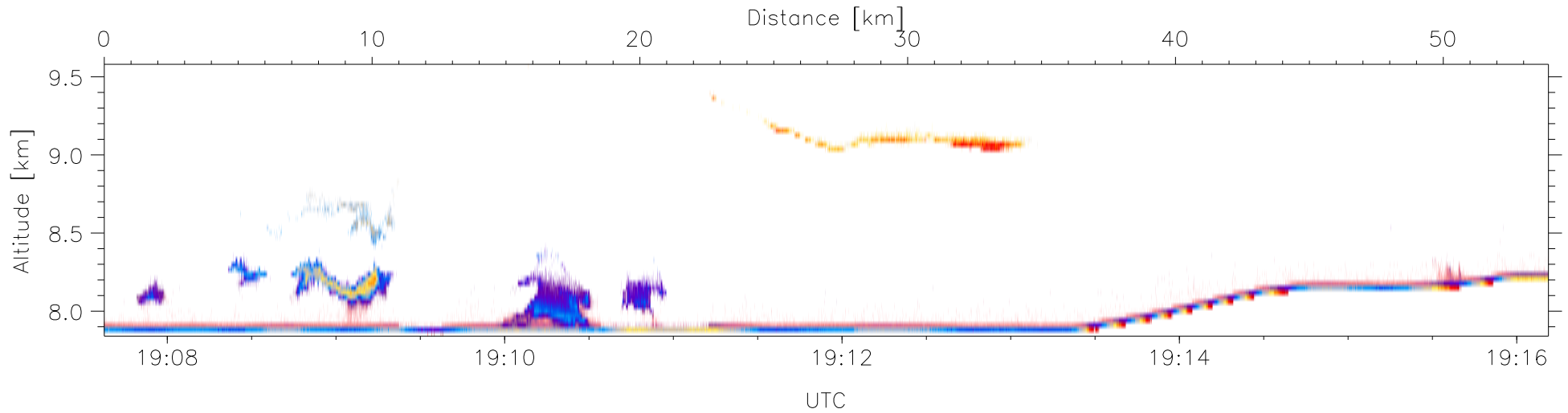
W2009-03-16-19-07-37: Up Reflectivity
